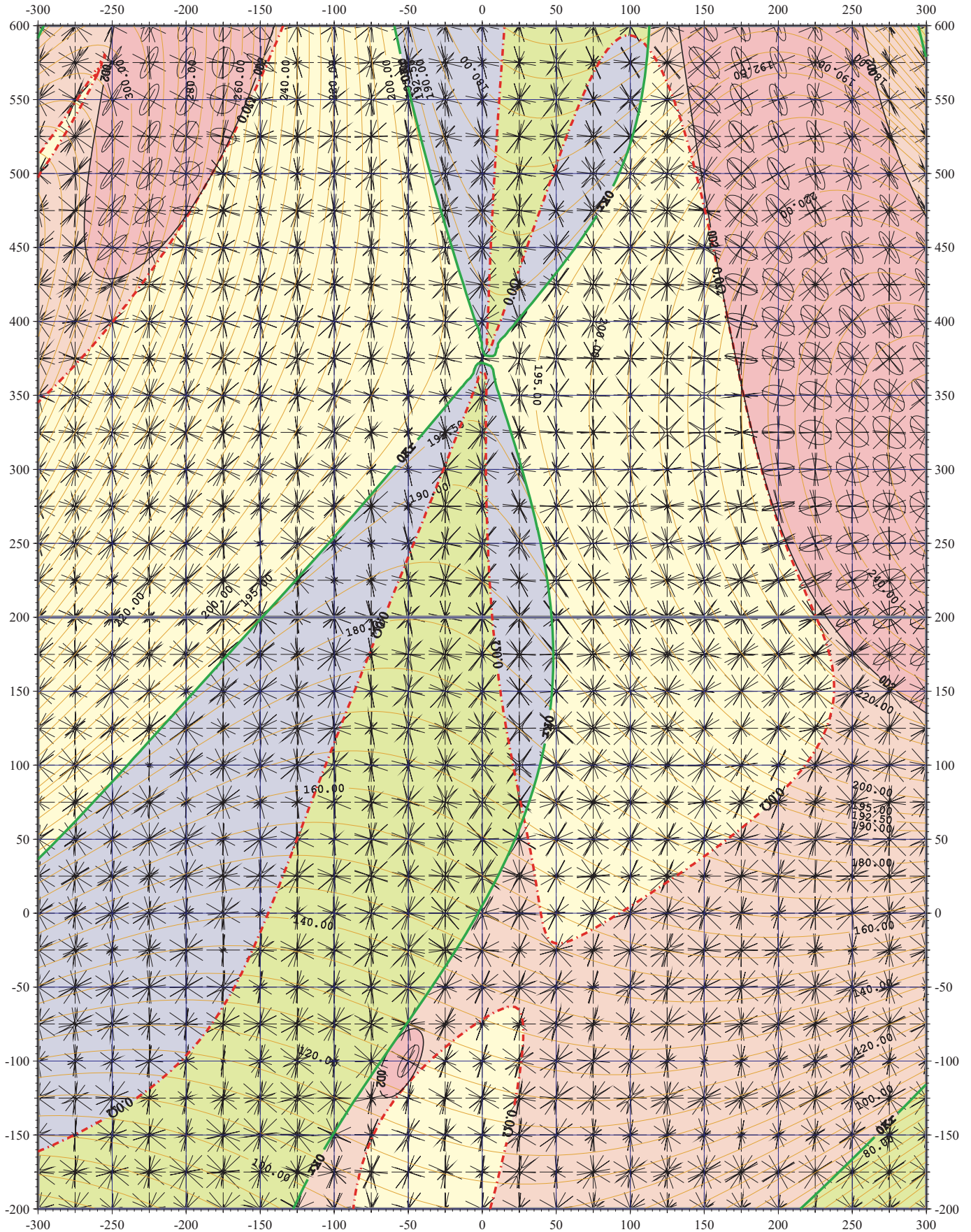
Grafická príloha 49.E Teoreticky presné „etalónové“ geometrické formy georeliéfu F_{XX} , F_{KX} , F_{KK} , F_{XX} dané do súvisu s priestorovým priebehom morfometrickej veličiny D_2 . K vrcholovému bodom štvorcovej siete sú priradené tvary Dupinovej idikatrix v závislosti od D_2 > 0 , D_2 < 0
